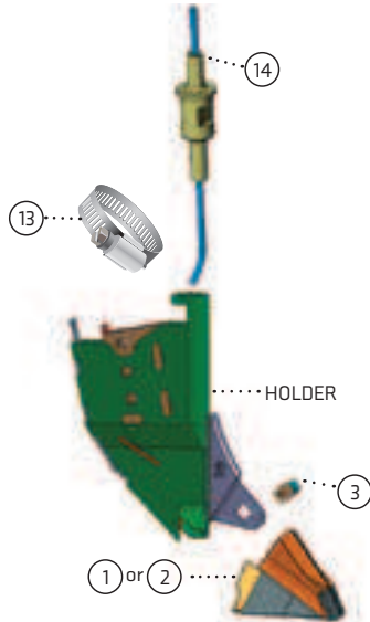
680-ASY-0711 680-ASY-0712 (SHOWN)
